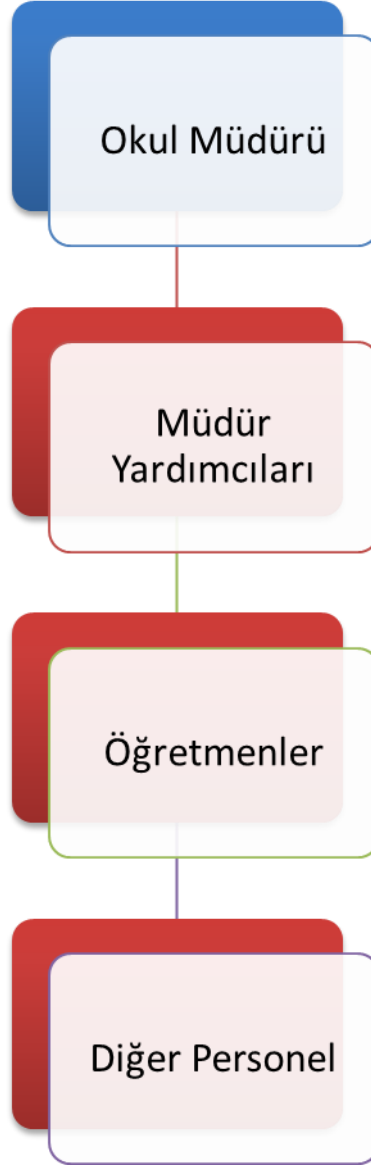
Şekil 10: Teşkilat Şeması
